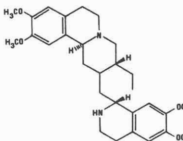
EMETINE
